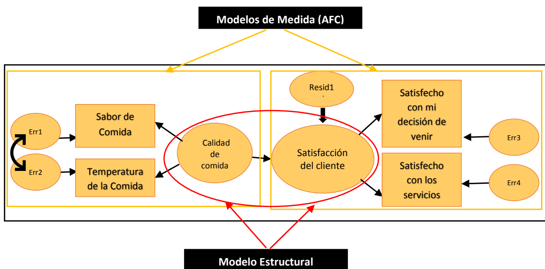
Gráfico No 17 Demarcación en Modelos de Medición y Modelo Estructural
