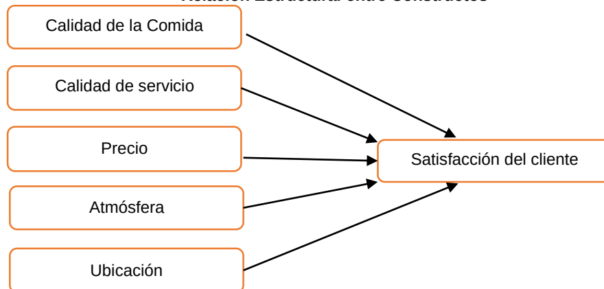
Gráfico No 14 Relación Estructural entre Constructos
