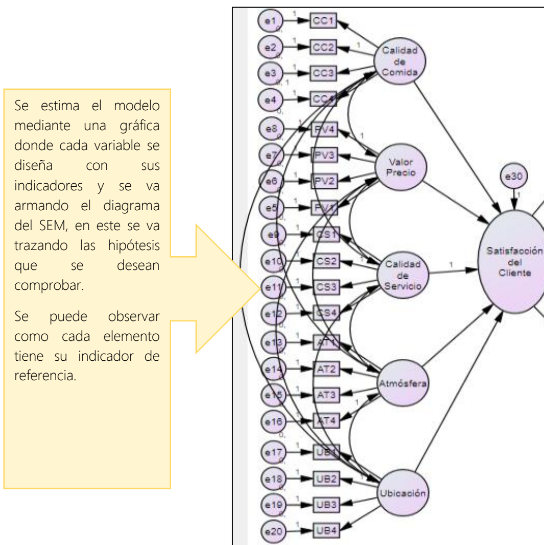
Gráfico No 24 Diagrama de la Estimación del Modelo
