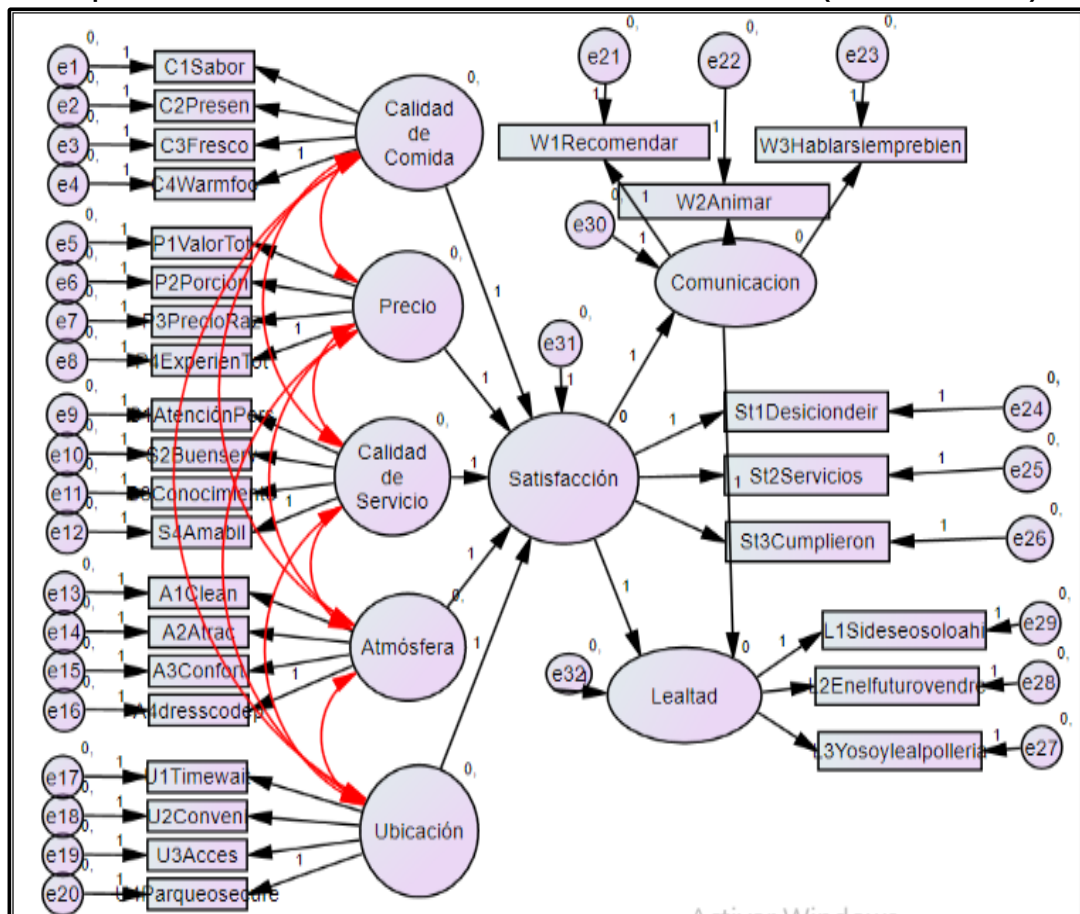
Gráfico No 25 Especificación del Modelo del Constructo de la Lealtad del cliente (No estandarizado)
