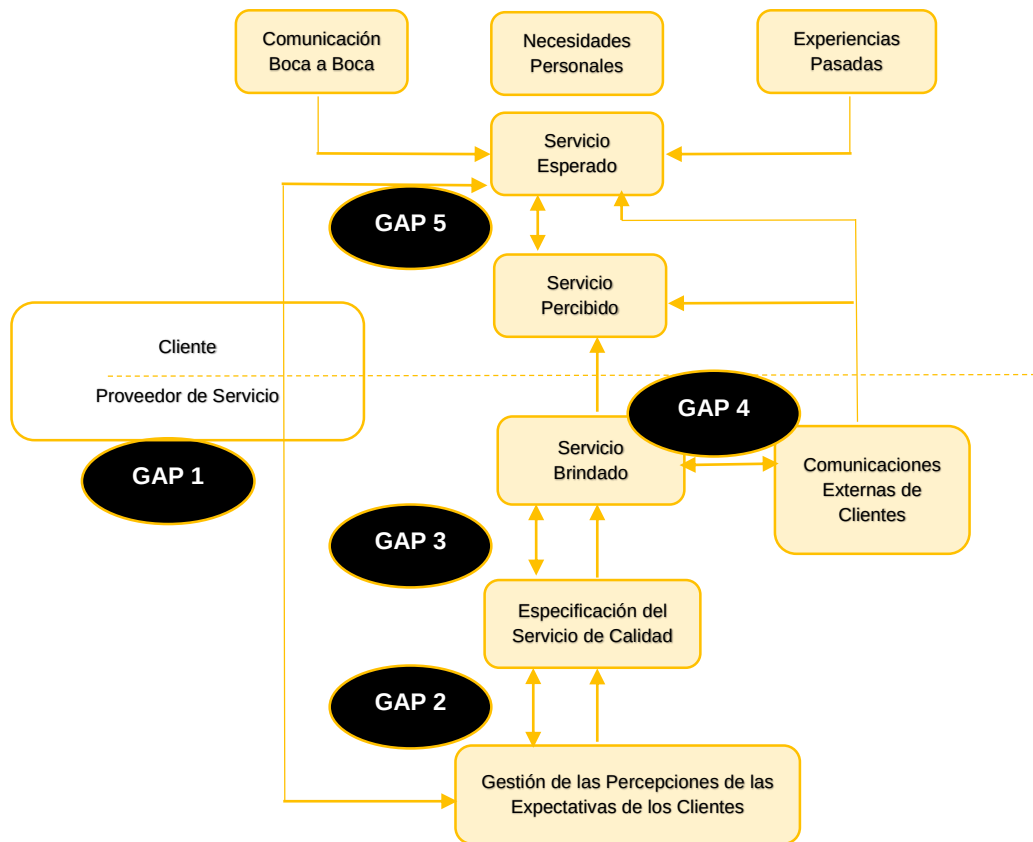
Gráfico No 9 Escala de Medición de la Calidad – SERVQUAL
