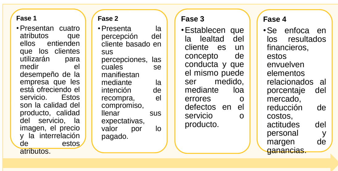
Gráfico No 11 Modelo de la Lealtad por Fases según Hoisington y Naumann
