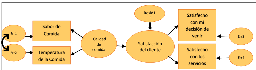
Gráfico No 16 Diagrama de Ruta
